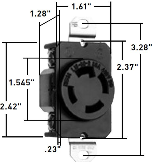
30A Receptacle
